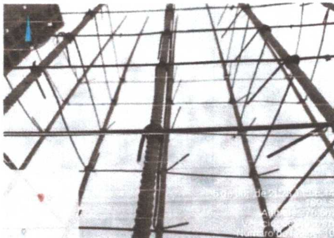
Foto 05 : pilar P39 com os estribos suplementares dobrados
