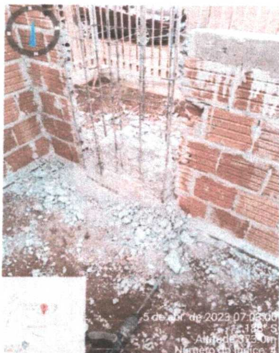
Foto 03 : pilar P39 completamente rompido
