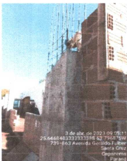
Foto 01: rompimento pilar P39
